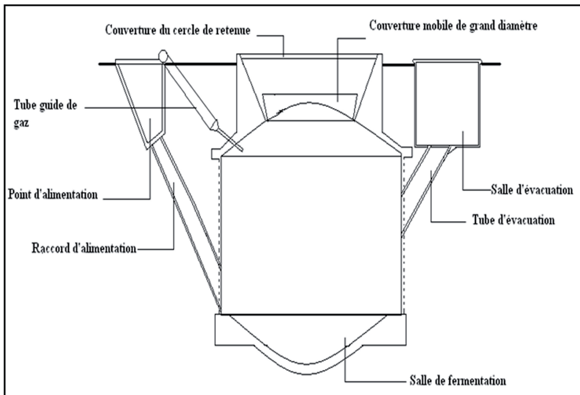
Figure 1: Schéma de principe et composants du digesteur rural de Sidi Thabet (Tunisie)
